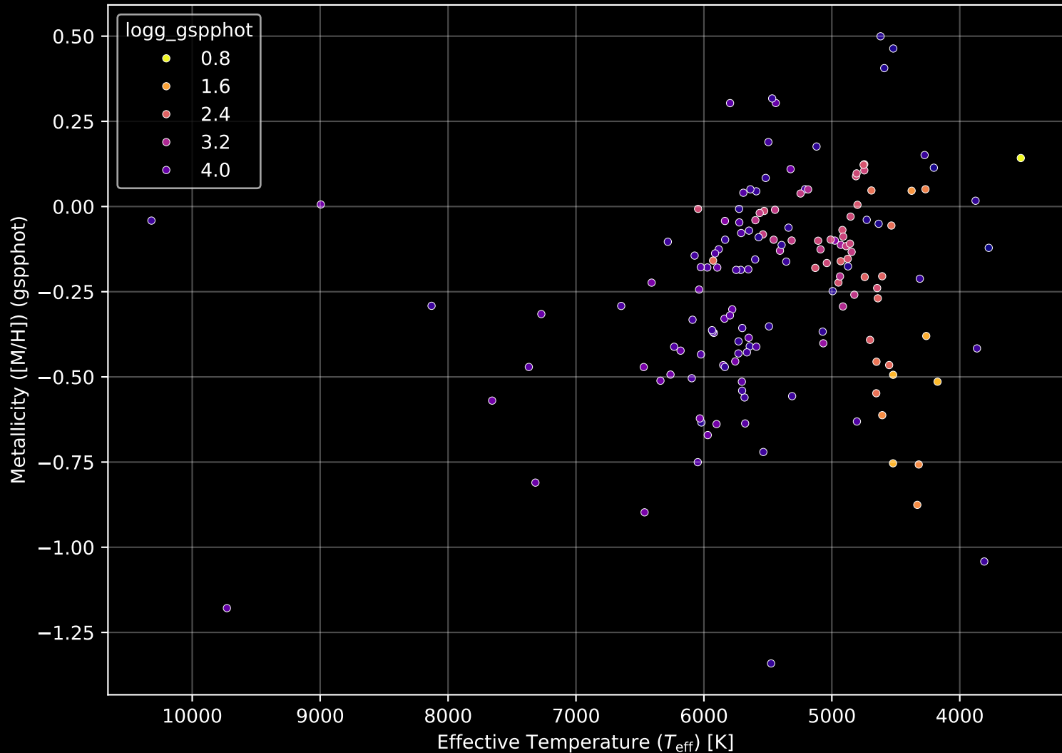
APOGEE DR17 Field: [274-23-O_TESS] Stellar Population Parameters (n= 155)
